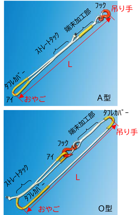
【O型・ループ吊り】
